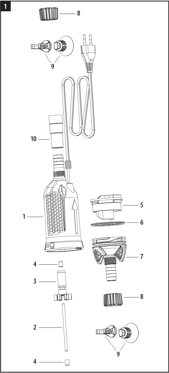
Fig. 1. UNI PUMP 1000/1500 – structure Rys. 1. Pompa UNI PUMP 1000/1500 – budowa Abb. 1. Pumpe UNI PUMP 1000/1500 – Aufbau Fig. 1. La pompe UNI PUMP 1000/1500 – la construction Рис. 1. Насос UNI PUMP 1000/1500 – комплектация Dib. 1. Bomba UNI PUMP 1000/1500 – estructura Fig. 1. La pompa pompa UNI 1000/1500 - Costruzione
